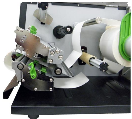
狹通道
